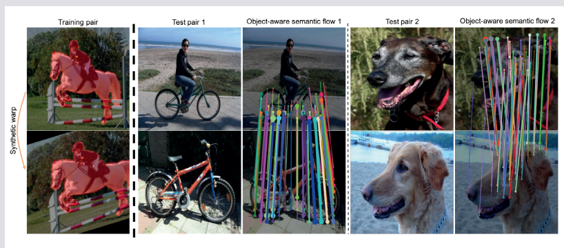
SFNET: Aprendiendo flujo semántico basado en el reconocimiento de objetos
